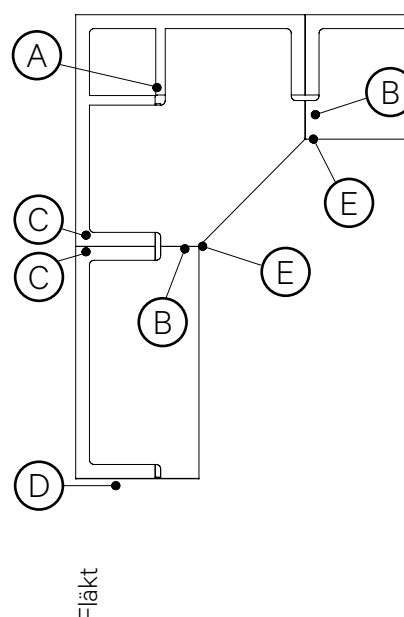
Exempelkök.
